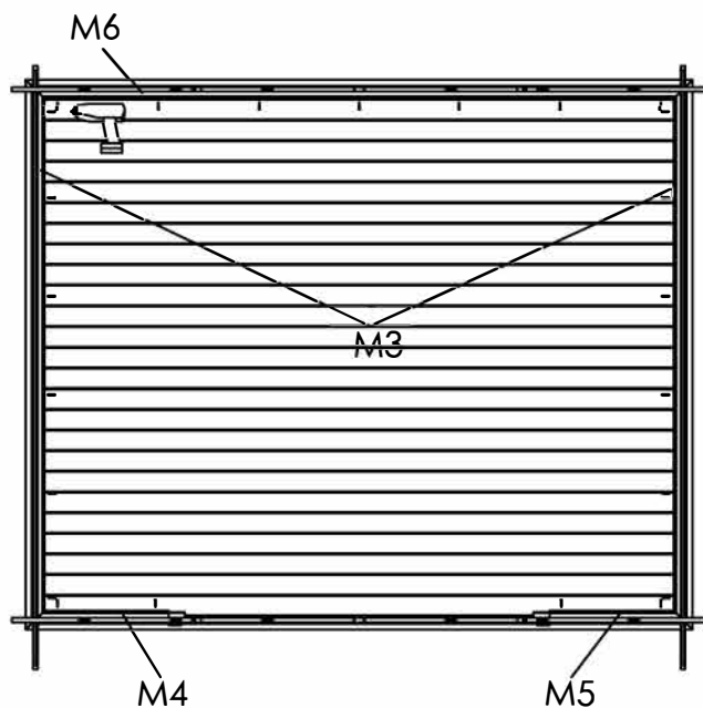
Element M3 - 2pcs Element M4 - 1pcs Element M5 - 1pcs Element M6 - 1pcs screws 3x40mm - 25 pcs
